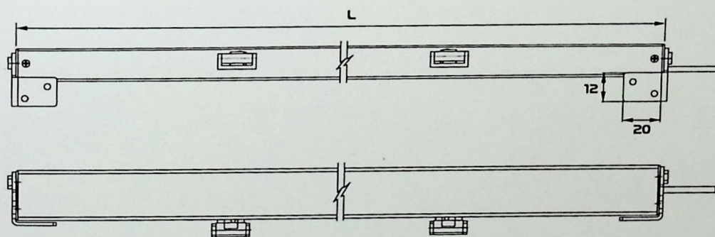
电动双链条式开窗器参数
