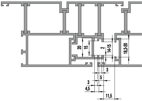
假中榫为对称型双C槽（外C槽安装主动扇锁座） 被动扇使用联动或分体式插销组件
