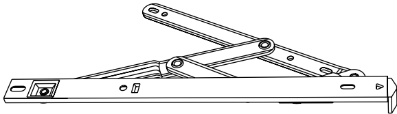
摩擦铰链
