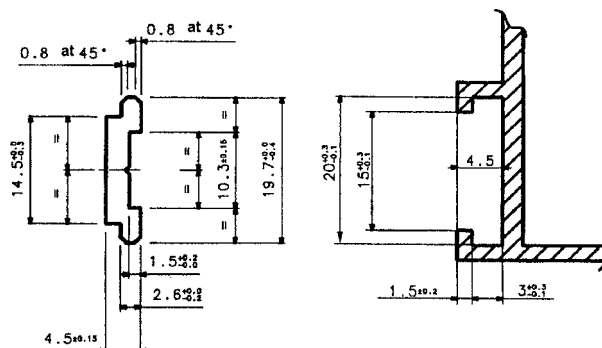
连接杆和型材的配合尺寸
