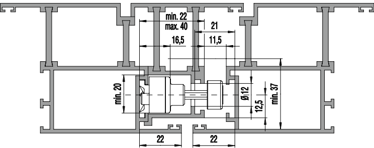
假中榫为单C槽（安装主动扇锁座） 被动扇使用可拆卸式7字形联动插销组件或分体式插销
