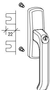
SPACIO 执手组件 - 带锁 2 个固定螺钉, 2 把钥匙 G-46554-96-R-*
