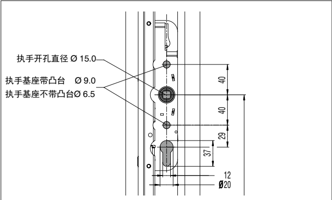
执手开孔样式
