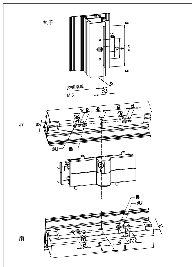
垂直中悬五金 UNITAS 88
