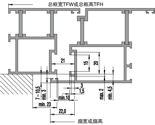
框和扇型材 扇为欧标槽口 15/20
