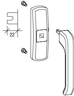
SPACIO 执手基座组件 2 个固定螺钉 C-46555-00-0-*
