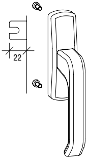
SPACIO 执手组件 - 不带锁 2 个固定螺钉 G-46551-00-0-*
