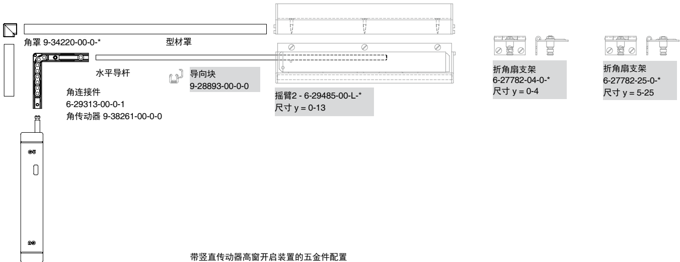
带竖直传动器高窗开启装置的五金件配置 根据摇臂数量的方案 1 到 3n
