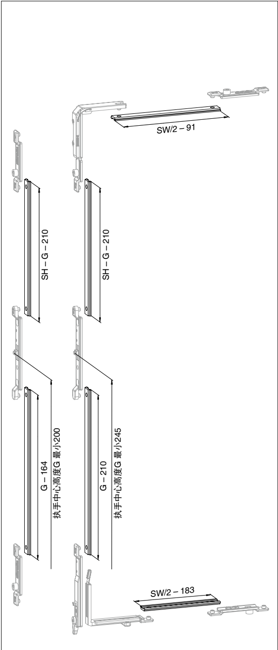
平开五金
