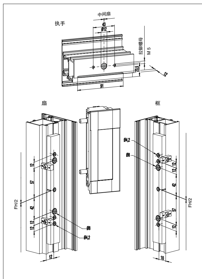
水平中悬五金 UNITAS 18/3
