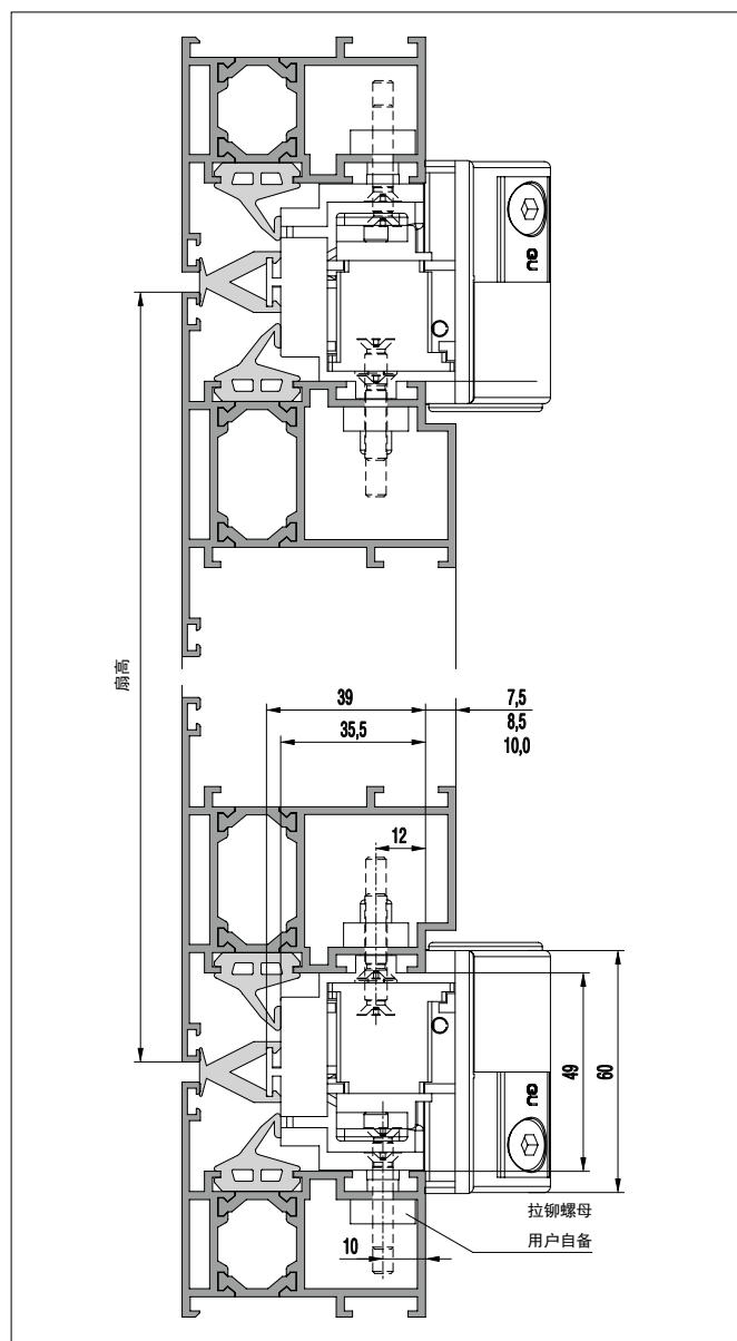
垂直中悬五金 UNITAS 88
