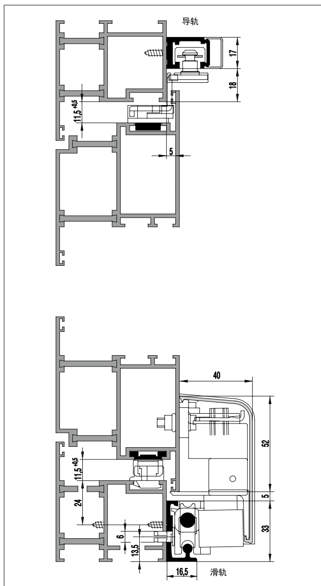
内倒侧滑系统 GU-968/150 mZ
