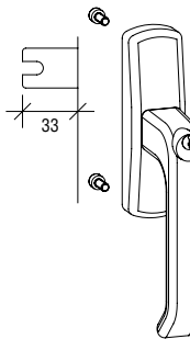
SPACIO 执手组件 - 带锁 2 个固定螺钉, 2 把钥匙 G-46597-96-0-*
