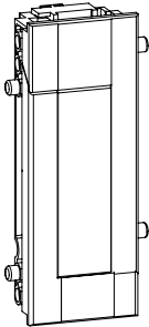
水平中悬合页 UNITAS 18/3
