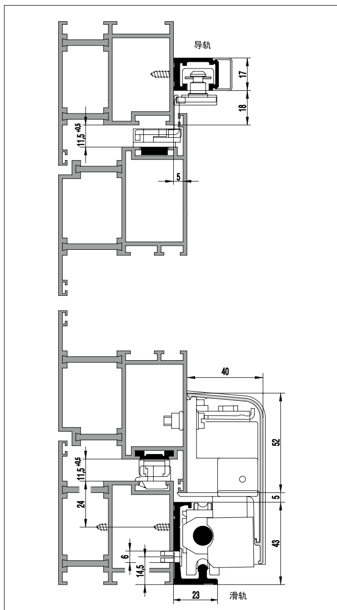
内倒侧滑系统 GU-968/200 mZ
