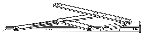
摩擦铰链
