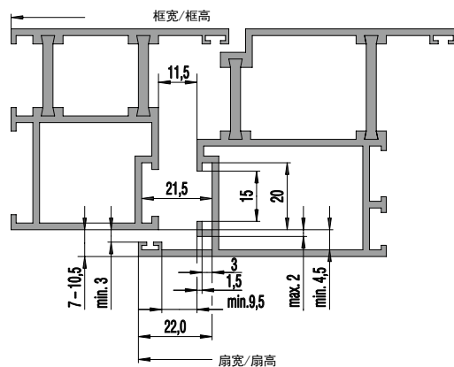
框扇型材欧标15/20槽
