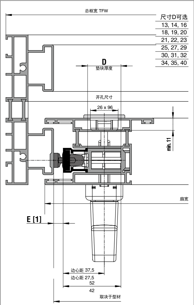
GU-934, GU-937 提升推拉传动器
