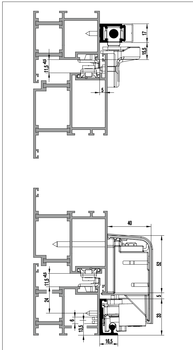
内倒侧滑系统 GU-90 oZ 具体配置请与G-U技术人员确认
