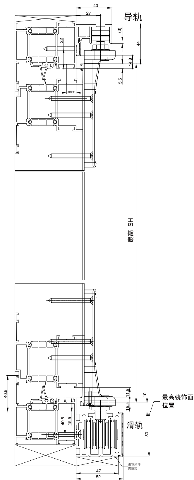
推拉折叠五金 GU-823
