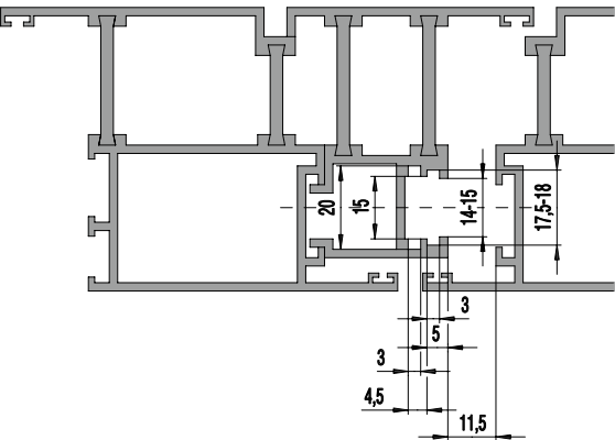
假中榫为双C槽（外C槽安装主动扇锁座） 被动扇使用联动或分体式插销组件
