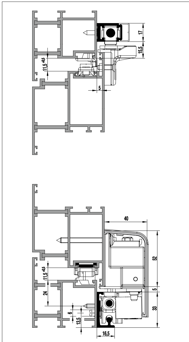
内倒侧滑系统 GU-968/150 oZ
