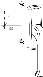
SPACIO 执手组件 - 不带锁 2 个固定螺钉 G-46595-96-0-*
