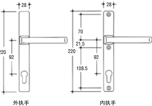
内外两面锁盖，锁盖宽度 28mm 内外执手（不带弹簧）
