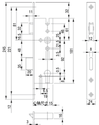
窄体锁 1314 方型不锈钢面板：3x24x245mm，方轴孔 8mm，中心距 92mm B 1314 000* *= 心轴尺寸 ( 边心距 )：1-25mm,2-30mm,3-35mm,4-40mm,5-45mm
