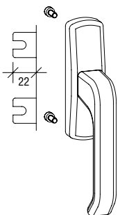
SPACIO 执手组件 - 不带锁 2 个固定螺钉 G-46552-96-R-*
