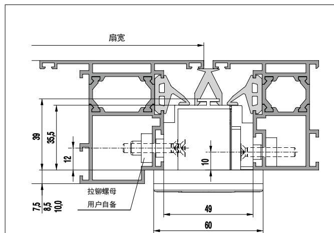
水平中悬五金 UNITAS 18/3
