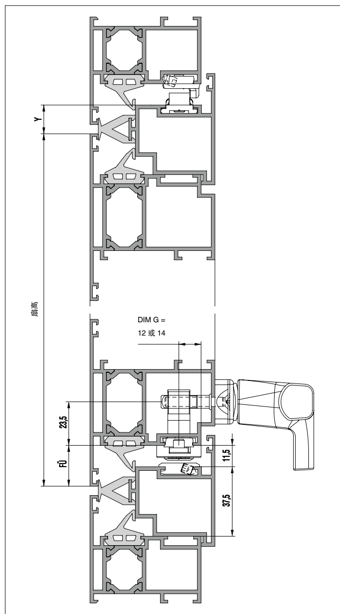
水平中悬五金 UNITAS 18/3
