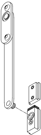
限位撑 K-13393-00-0-1
