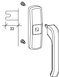
SPACIO 执手基座组件 2 个固定螺钉 C-46596-96-0-* 可拆卸式SPACIO手柄 C-18888-00-0-*
