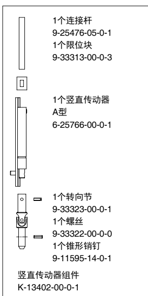
带竖直传动器高窗开启装置的五金件配置 根据摇臂数量的方案 1 到 3n
