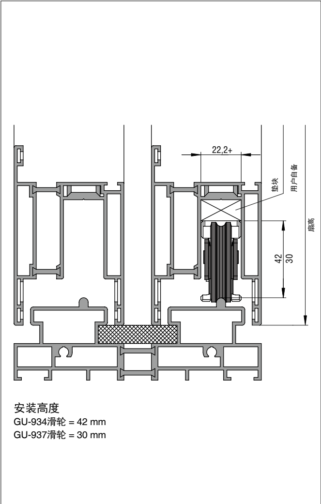
GU-934, GU-937 滑轮
