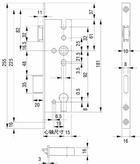
窄体锁 1300 方型不锈钢面板：3x16x255mm，方轴孔 8mm，中心距 92mm B 1300 000* *= 心轴尺寸 ( 边心距 )：1-25mm,2-30mm,3-35mm,4-40mm,5-45mm
