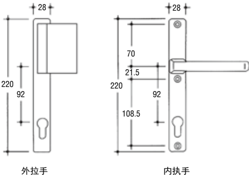
外部拉手盖和内锁盖 - 锁盖宽度 28mm 1 个外部拉手，1 个内执手（不带弹簧）
