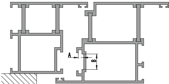
角传动器 6-30889-00-0-1 欧标槽口 15/20 欧标深槽 15/20, 尺寸A=最大3.9mm, 尺寸B=最大13mm, 6-30889-01-0-1 欧标深槽 15/20 尺寸A=4.0-5.1mm
