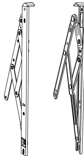
摩擦铰链 上悬窗
