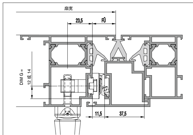
垂直中悬五金 UNITAS 88
