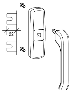
SPACIO 执手基座组件 2 个固定螺钉 C-46556-96-R-* 可拆卸式SPACIO手柄 C-18888-00-0-*
