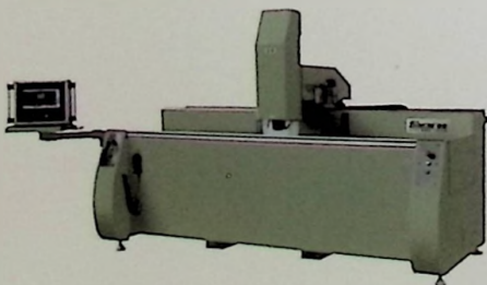
GCGZA-CNC-3000 铝型材数控四轴加工中心 CNC Four-axis Machining Center for Aluminum Profiles
