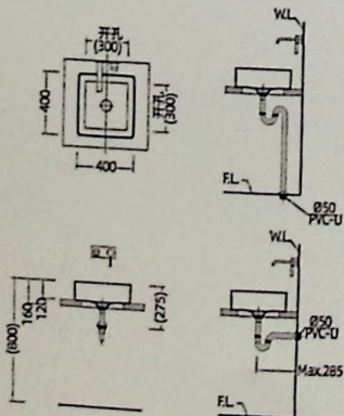
安装尺寸图
