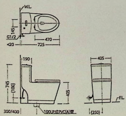
安装尺寸图
