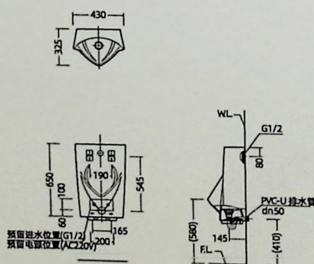
安装尺寸图
