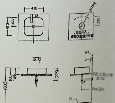
安装尺寸图
