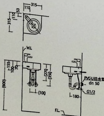
安装尺寸图
