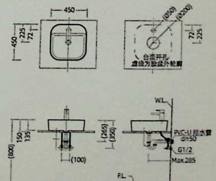
安装尺寸图
