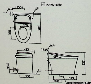
安装尺寸图
