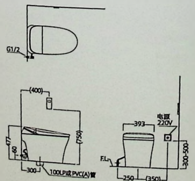
安装尺寸图
