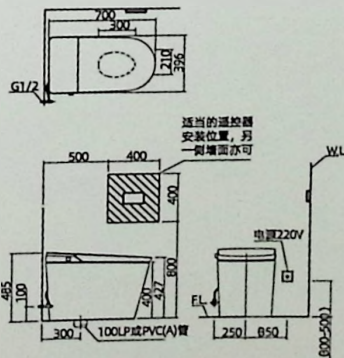
安装尺寸图
