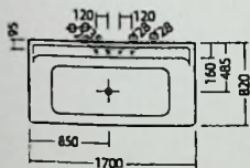
安装尺寸图
