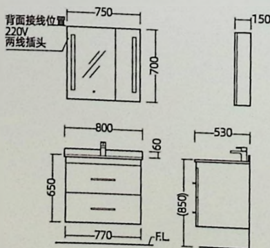
安装尺寸图
