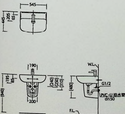
安装尺寸图
