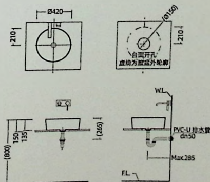
安装尺寸图
