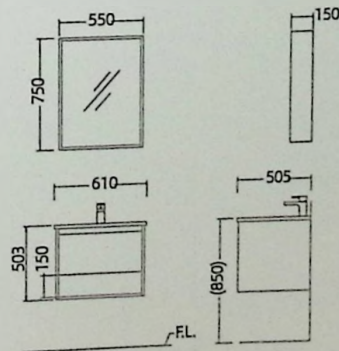
安装尺寸图
