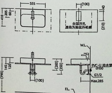
安装尺寸图
