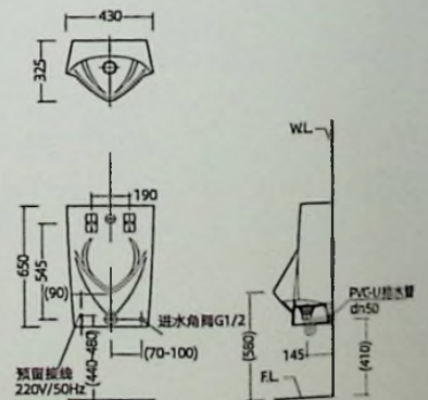
安装尺寸图
