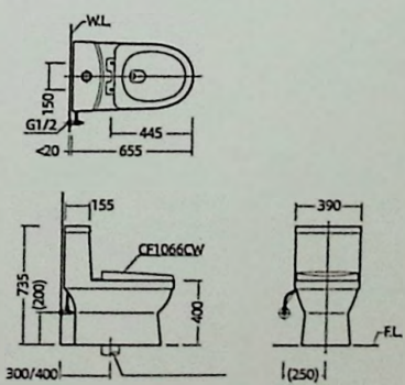
安装尺寸图
