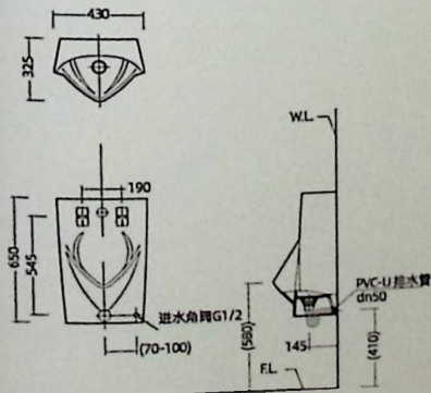
安装尺寸图
