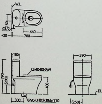
安装尺寸图
