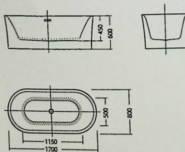
安装尺寸图
