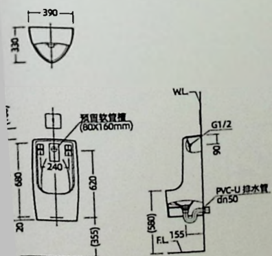
安装尺寸图
