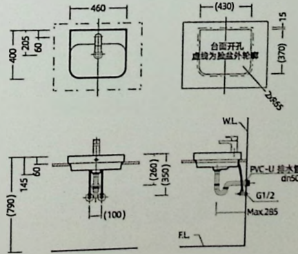
安装尺寸图
