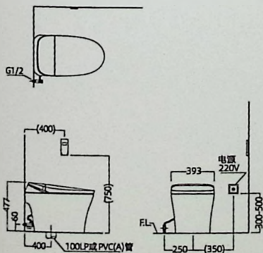
安装尺寸图
