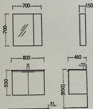
安装尺寸图
