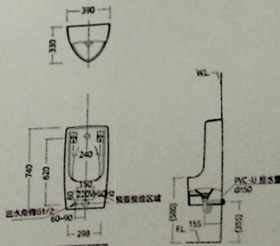
安装尺寸图
