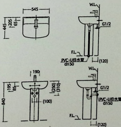
安装尺寸图
