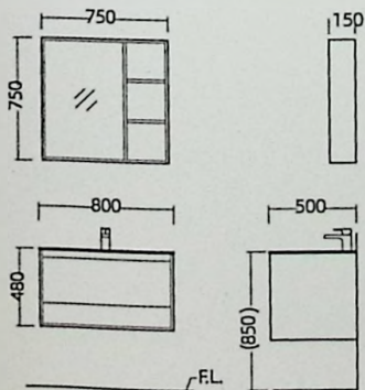
安装尺寸图
