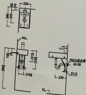
安装尺寸图
