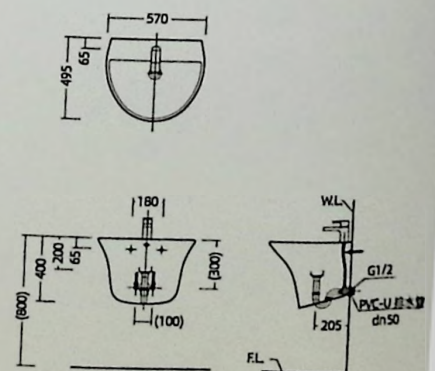
安装尺寸图
