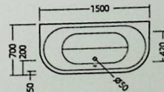
安装尺寸图
