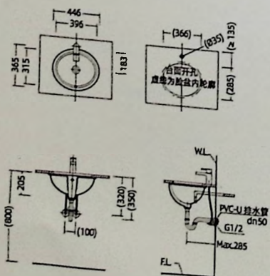
安装尺寸图
