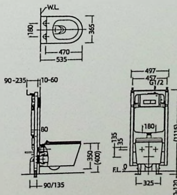
安装尺寸图
