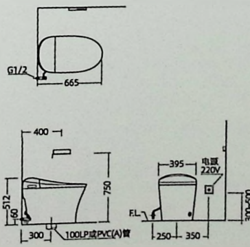
安装尺寸图
