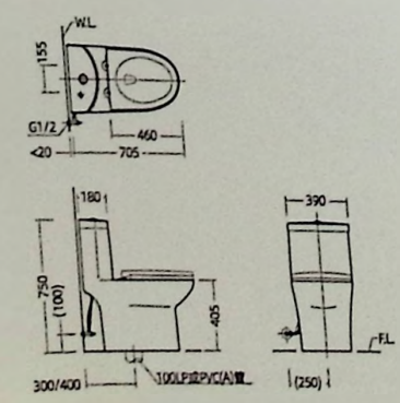
安装尺寸图
