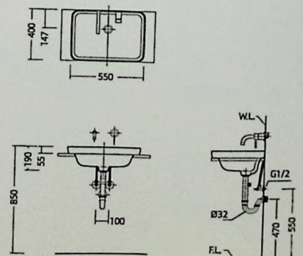
安装尺寸图
