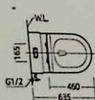
安装尺寸图
