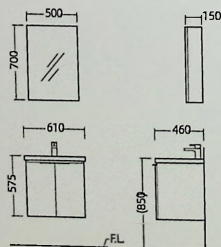
安装尺寸图
