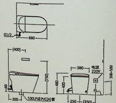
安装尺寸图
