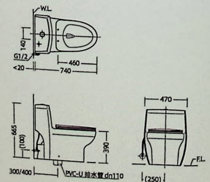
安装尺寸图
