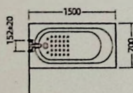
安装尺寸图
