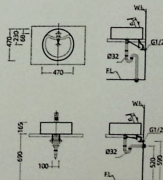
安装尺寸图
