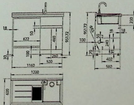
安装尺寸图
