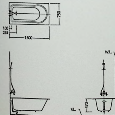
安装尺寸图
