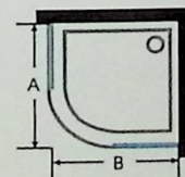
安装尺寸图
