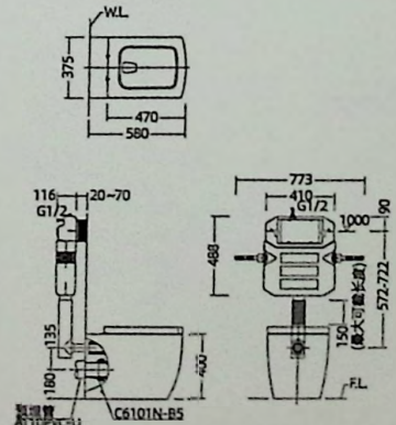
安装尺寸图
