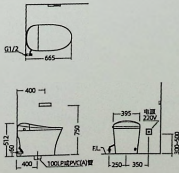
安装尺寸图
