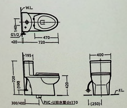
安装尺寸图
