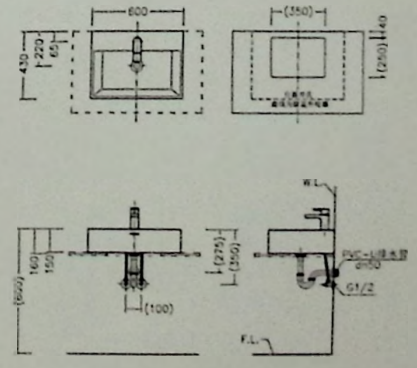
安装尺寸图
