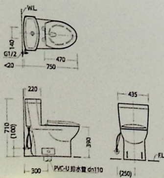
安装尺寸图
