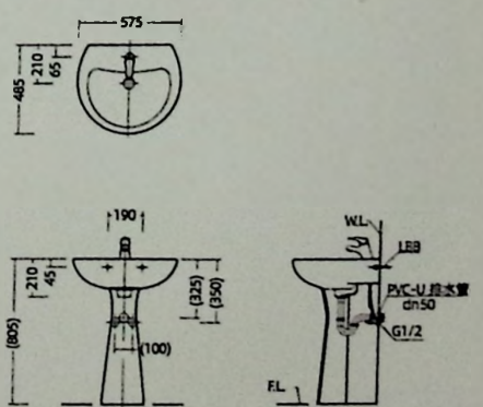
安装尺寸图
