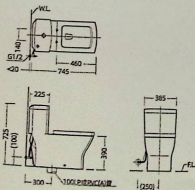
安装尺寸图
