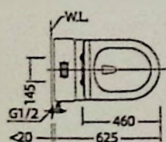
安装尺寸图
