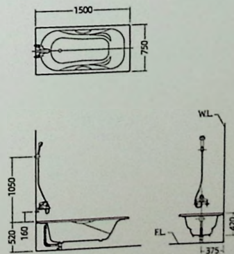
安装尺寸图
