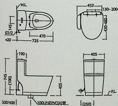
安装尺寸图
