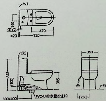
安装尺寸图
