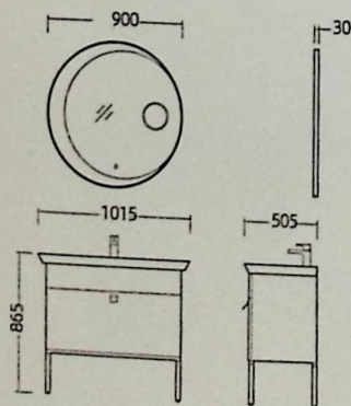
安装尺寸图
