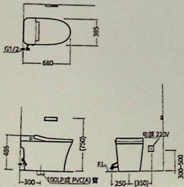
安装尺寸图
