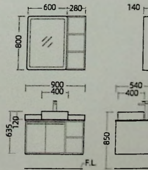
安装尺寸图
