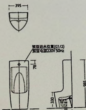
安装尺寸图
