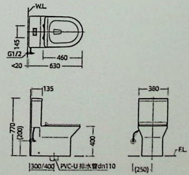
安装尺寸图
