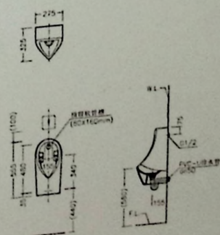
安装尺寸图
