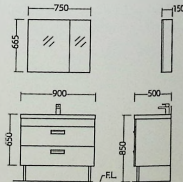
安装尺寸图
